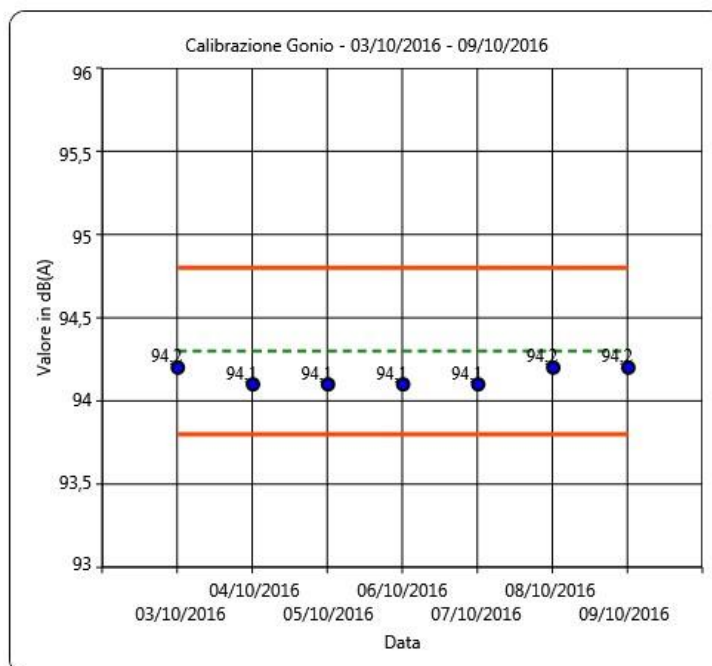
Figura 30: Calibrazioni check postazione Gonio
