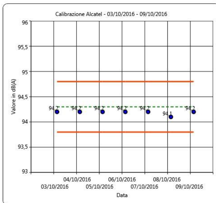
Figura 31: Calibrazioni check postazione Alcatel
