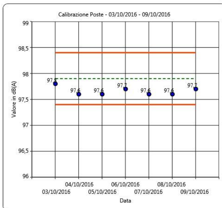
Figura 29: Calibrazioni check postazione Poste
