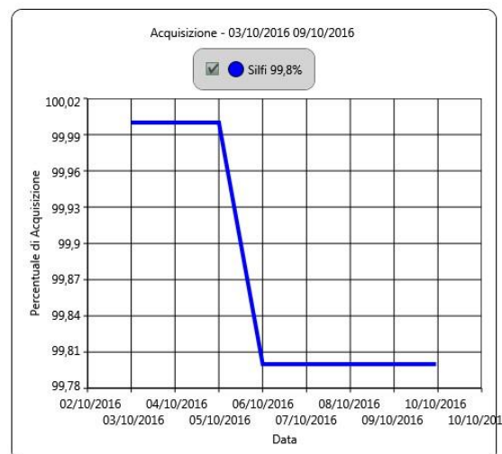
Figura 25: Percentuale di acquisizione settimanale della postazione Silfi
