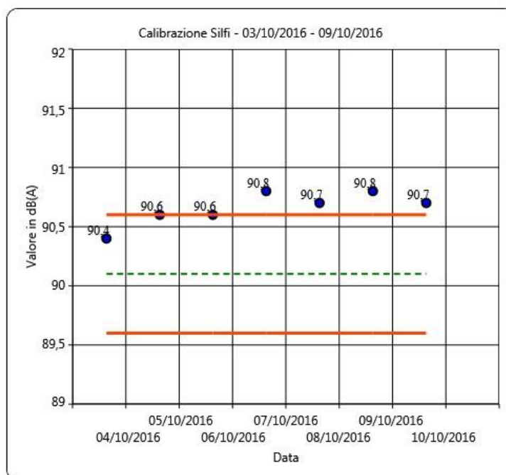
Figura 28: Calibrazioni check postazione Silfi
