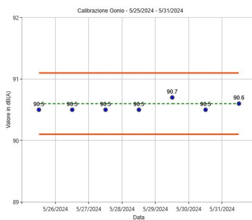
Figura 28: Calibrazioni check postazione Gonio
