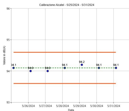
Figura 29: Calibrazioni check postazione Alcatel
