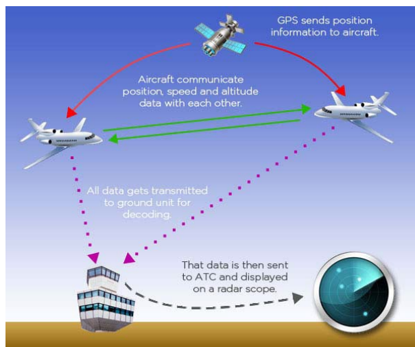
Figura 28: Il sistema ADS-B
