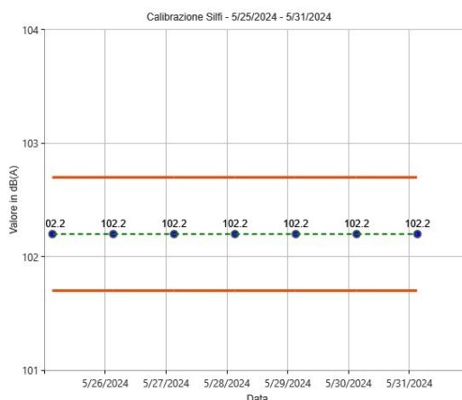
Figura 26: Calibrazioni check postazione Sil i
