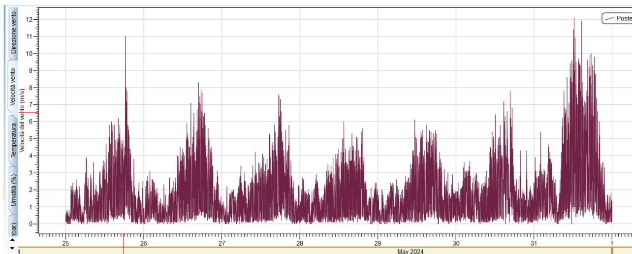
Figura 21: Grafico della velocità del vento acquisita dalla centralina POSTE
