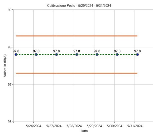
Figura 27: Calibrazioni check postazione Poste
