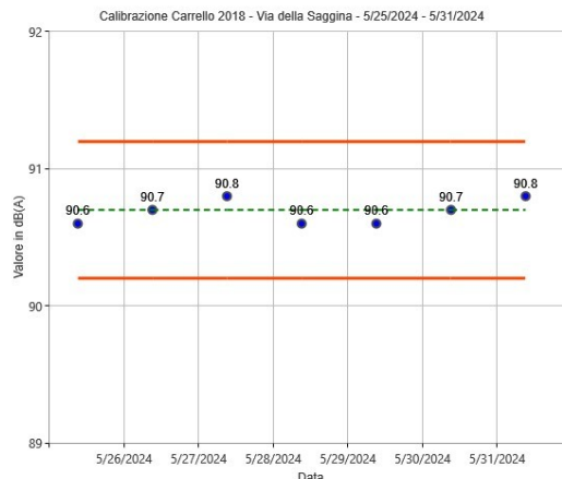
Figura 30: Calibrazioni check postazione Carrello 2018 Via della Saggina
