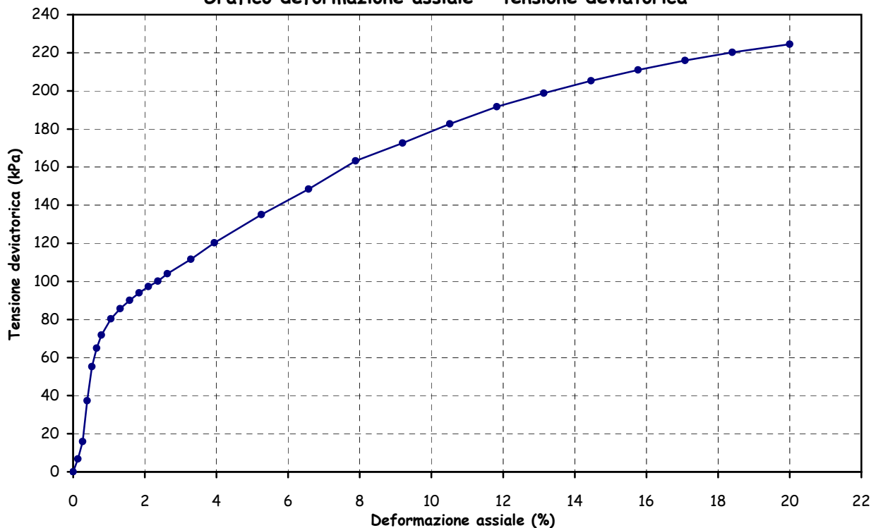
Grafico deformazione assiale - tensione deviatorica
