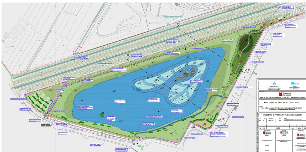
Figura 11 – Estratto Tav.FLR-MPL-PFTE-CAP3-005-PA-PL_S Croce Plan Sez Prog L'area di Santa Croce
