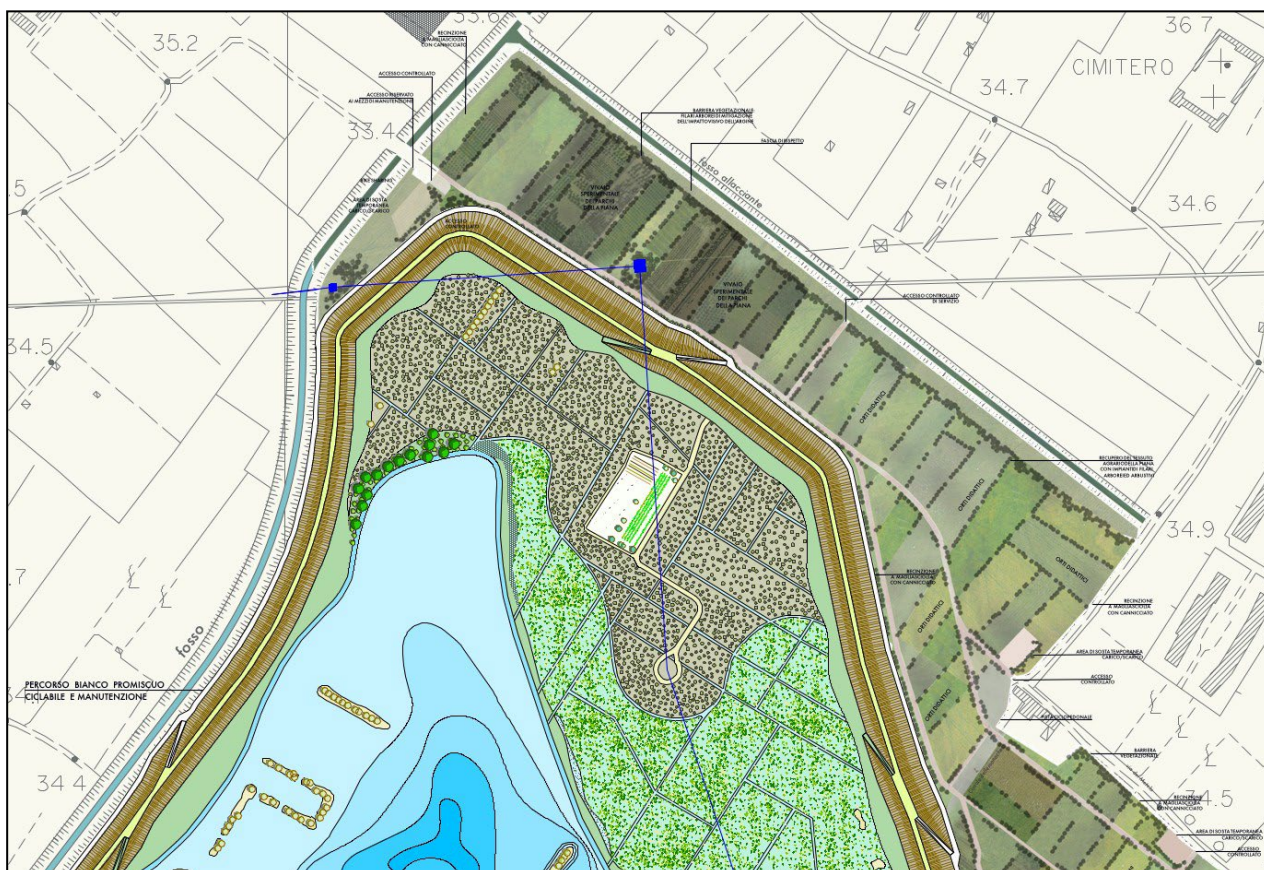
Figura 5.4 – Planimetria del progetto del parco Didattico e Vivaio Sperimentale
