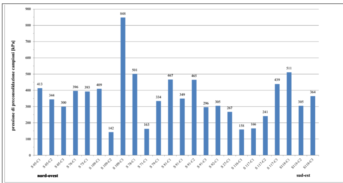
Figura 9 - Valori della pressione di preconsolidazione ottenuti dalle prove di laboratorio eseguite sui campioni prelevati dai sondaggi realizzati all'interno delle diverse aree del sistema della viabilità e di aree circostanti del sedime aeroportuale, con i campioni posizionati da nord-ovest (a sinistra, nel grafico) a sud-est (a destra, nel grafico).
