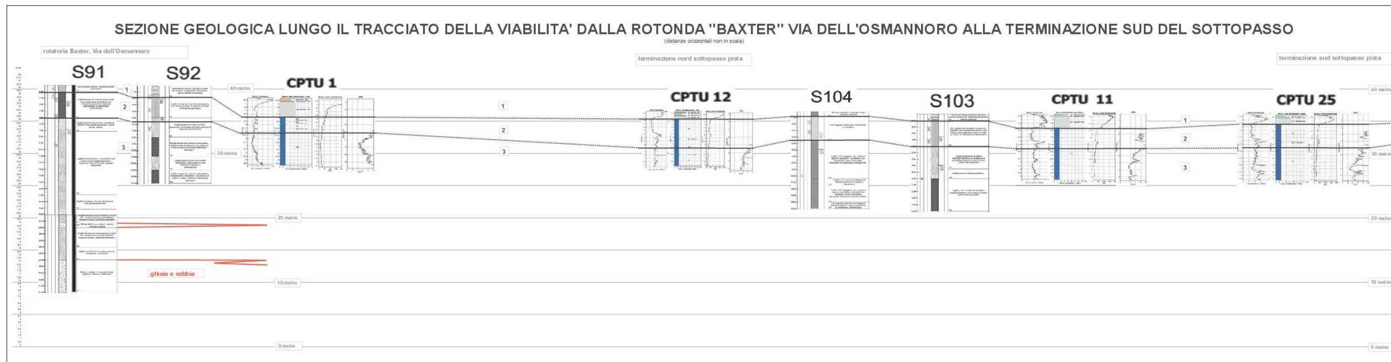
Figura 7 - Sezione geologica tracciato viabilità dalla rotonda B "BAXTER" via dell'Osmannoro alla terminazione sud del sottoattraversamento pista.
