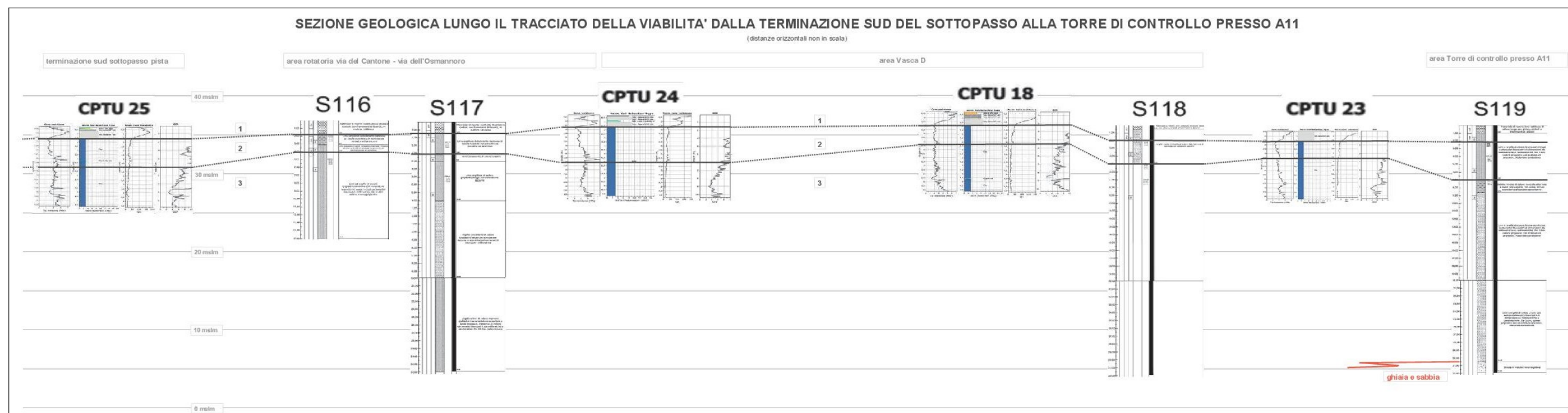
Figura 8 - Sezione geologica tracciato viabilità dalla terminazione sud del sottoattraversamento pista alla torre di controllo presso Autostrada A11.
