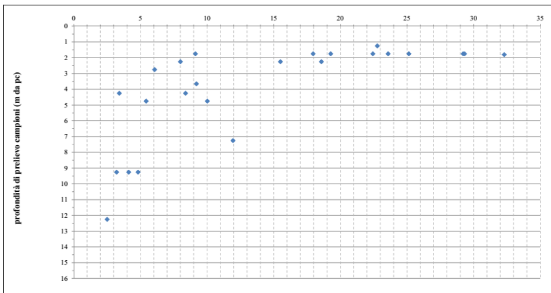
Figura 11 - Valori di OCR in funzione della profondità di prelievo (m dal p.c.), ottenuti dalle prove di laboratorio eseguite sui campioni dei sondaggi realizzati per la presente relazione e di altre aree del sedime aeroportuale.
