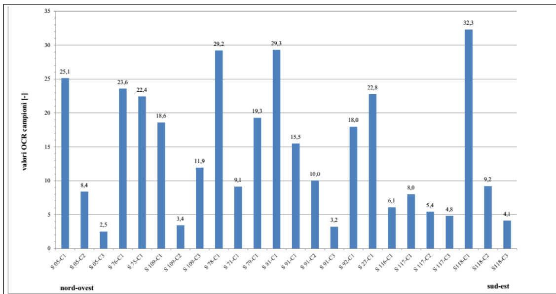
Figura 10 - Valori di OCR ottenuti dalle prove di laboratorio eseguite sui campioni prelevati dai sondaggi realizzati all'interno delle diverse aree oggetto della presente relazione e di altre circostanti del sedime aeroportuale, con i campioni posizionati da nord-ovest (a sinistra, nel grafico) a sud-est (a destra, nel grafico).
