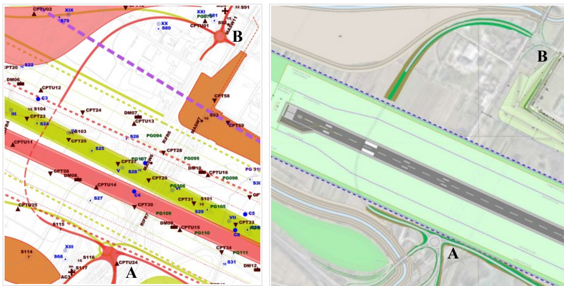
Figura 6 - Tratto viabilità compresa fra le due rotonde A e B con il sottoattraversamento della pista
