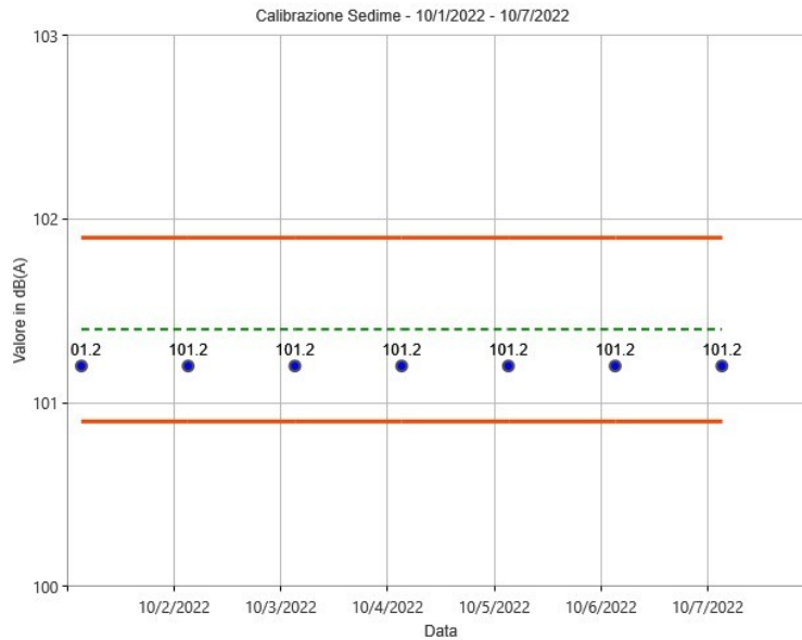
Figura 27: Calibrazioni check postazione Zona Militare Sedime
