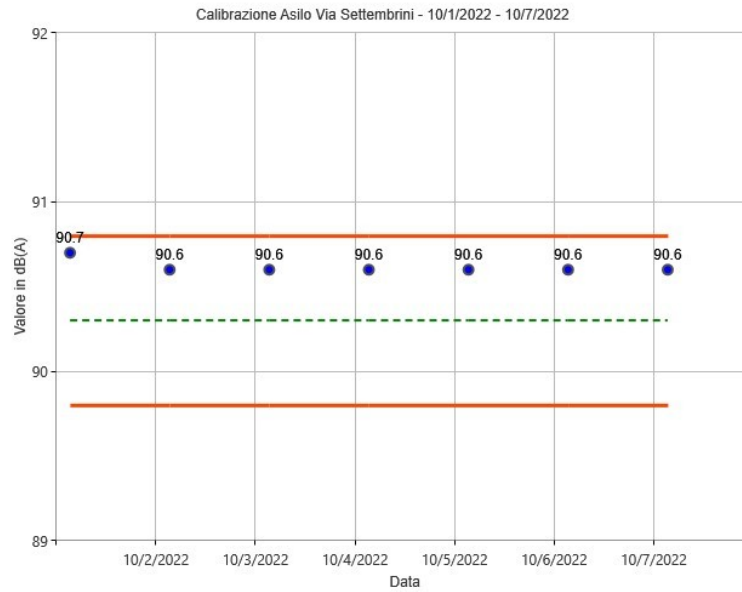
Figura 25: Calibrazioni check postazione Asilo Via Settembrini
