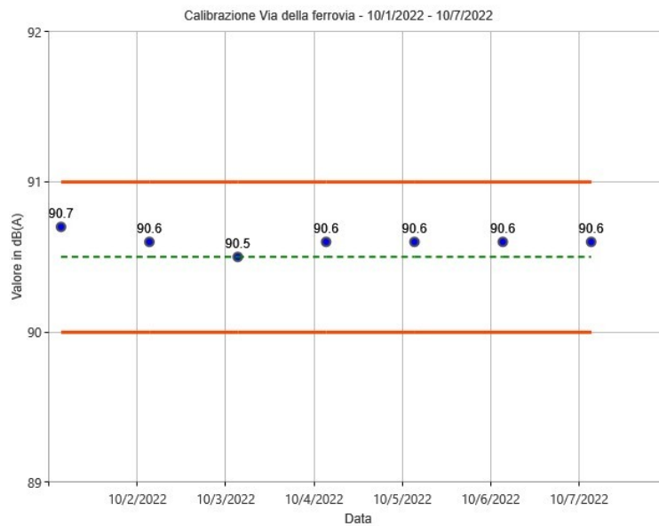
Figura 26: Calibrazioni check postazione Via della Ferrovia
