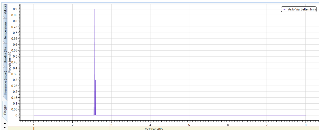
Figura 22: Grafico della pioggia acquisita dalla centralina Asilo Via Settembrini per il periodo 1 7 ottobre 2022
