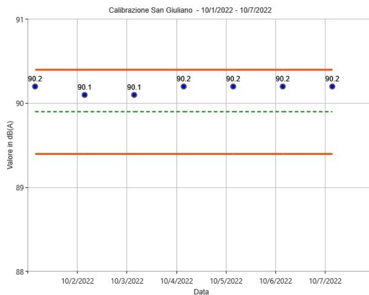
Figura 28: Calibrazioni check postazione San Giuliano
