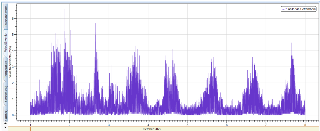
Figura 21: Grafico della velocità del vento acquisita dalla centralina Asilo Via Settembrini per il periodo 1 7 ottobre 2022
