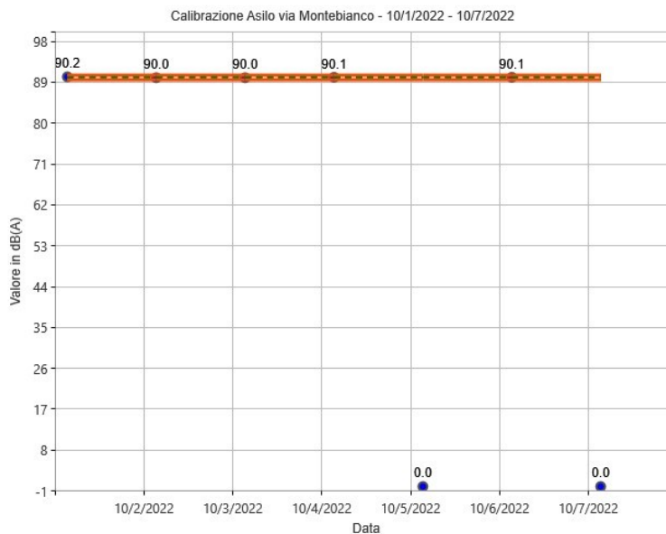
Figura 24: Calibrazioni check postazione Asilo Via Monte Bianco
