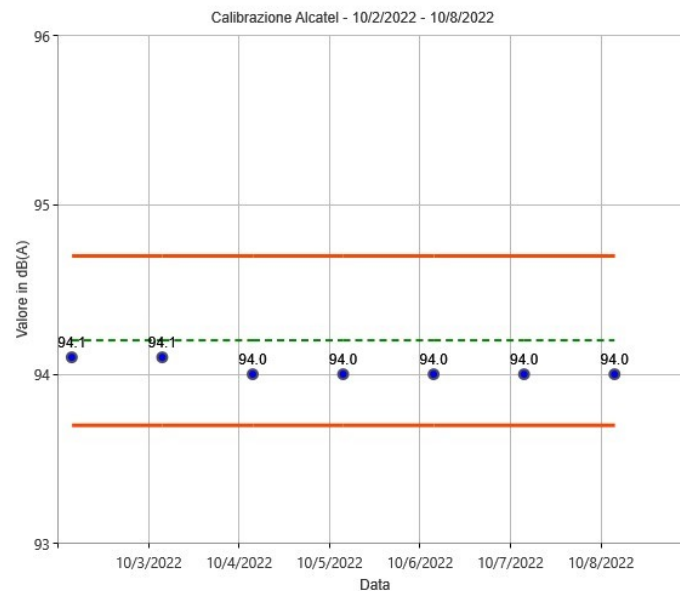
Figura 27: Calibrations check postazione Alcatel
