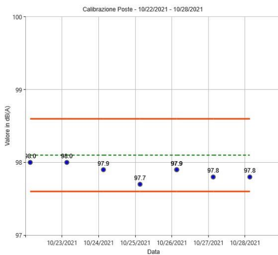
Figura 25: Calibrazioni check postazione Poste
