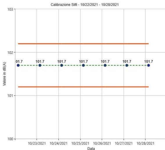
Figura 24: Calibrazioni check postazione Silfi
