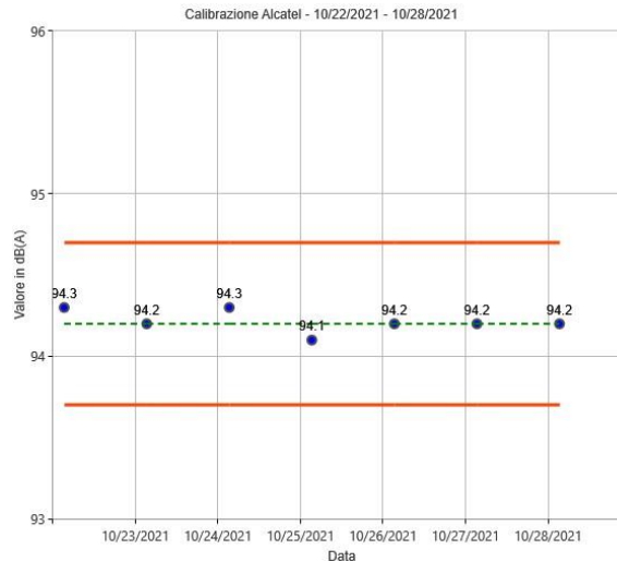
Figura 27: Calibrazioni check postazione Alcatel
