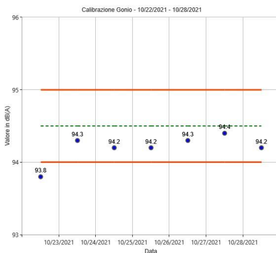
Figura 26: Calibrazioni check postazione Gonio
