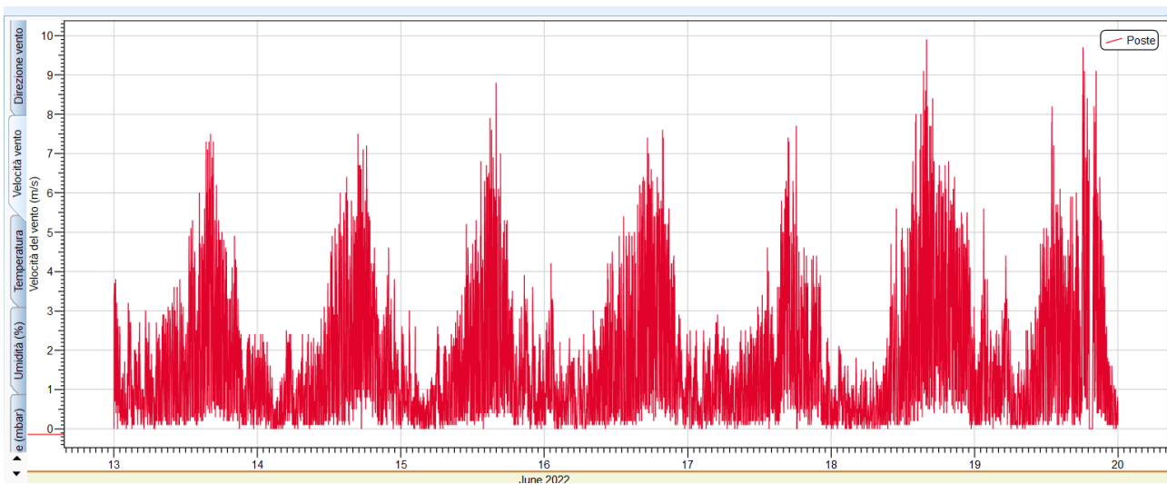
Figura 19: Grafico della velocità del vento acquisita dalla centralina POSTE
