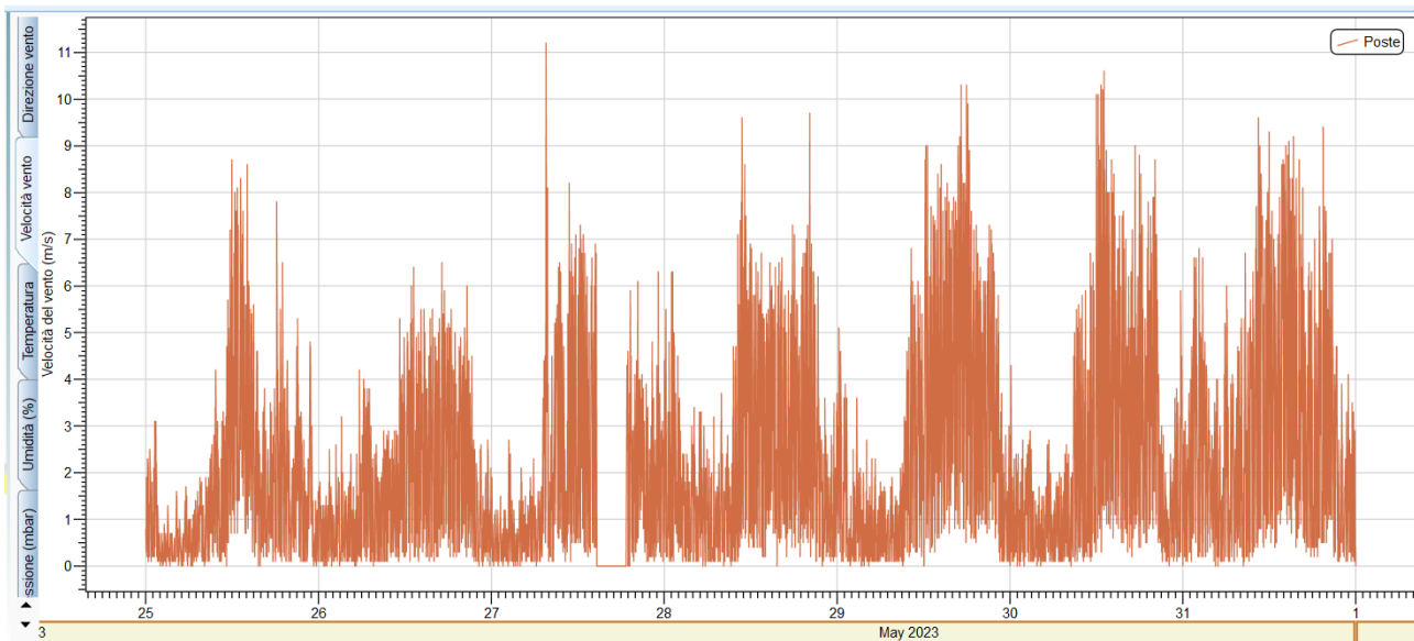
Figura 19: Grafico della velocità del vento acquisita dalla centralina POSTE
