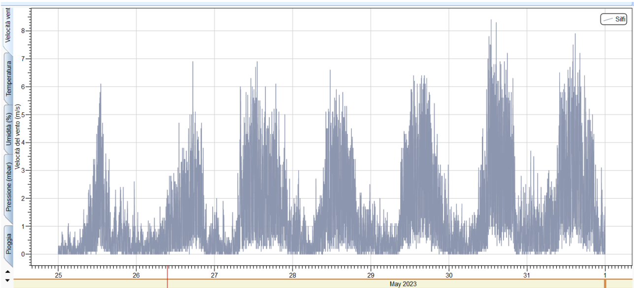
Figura 21: Grafico della velocità del vento acquisita dalla centralina Silfi
