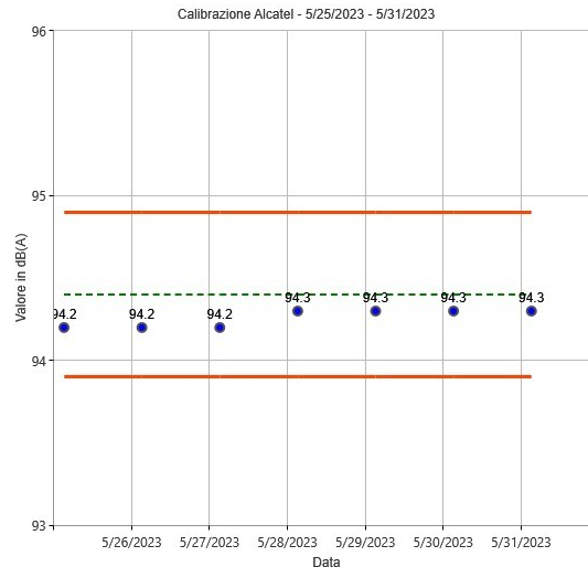
Figura 27: Calibrazioni check postazione Alcatel
