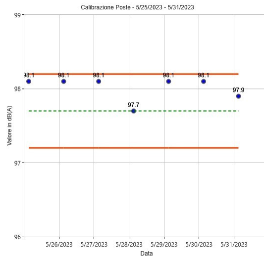
Figura 25: Calibrazioni check postazione Poste
