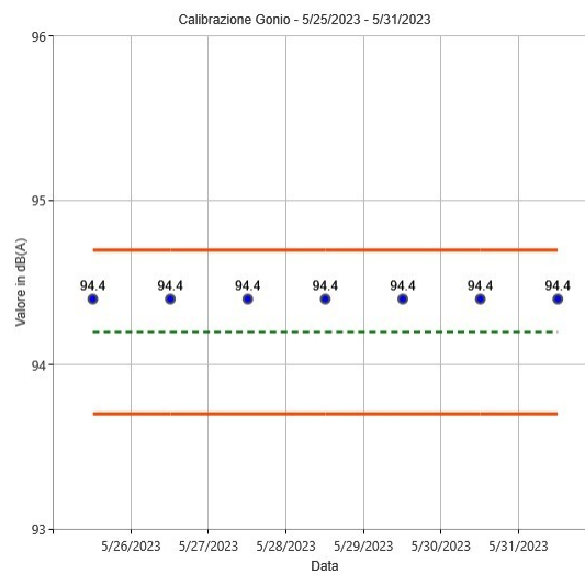
Figura 26: Calibrazioni check postazione Gonio
