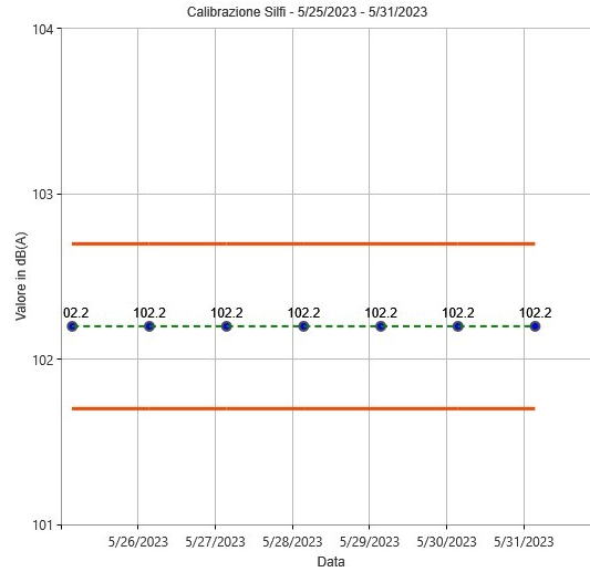
Figura 24: Calibrazioni check postazione Silfi
