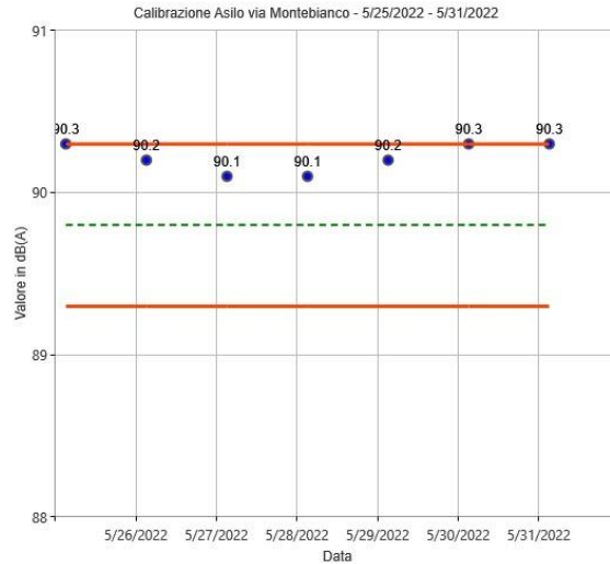
Figura 24: Calibrazioni check postazione Asilo Via Monte Bianco
