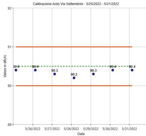
Figura 25: Calibrazioni check postazione Asilo Via Settembrini
