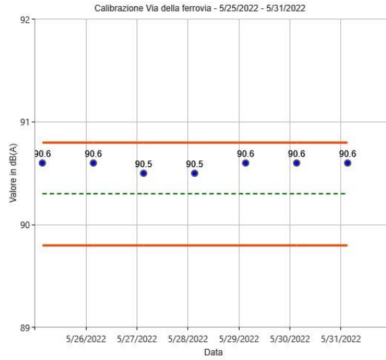
Figura 26: Calibrazioni check postazione Via della Ferrovia
