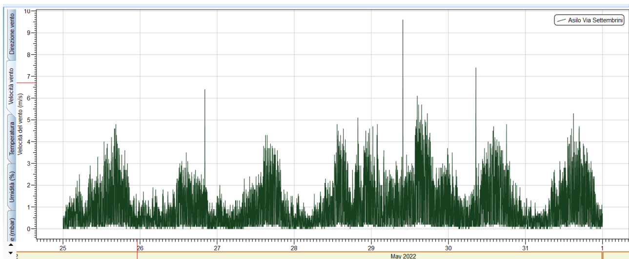
Figura 21: Grafico della velocità del vento acquisita dalla centralina Asilo Via Settembrini per il periodo 25-31 maggio 2022
