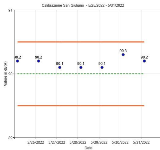
Figura 28: Calibrazioni check postazione San Giuliano
