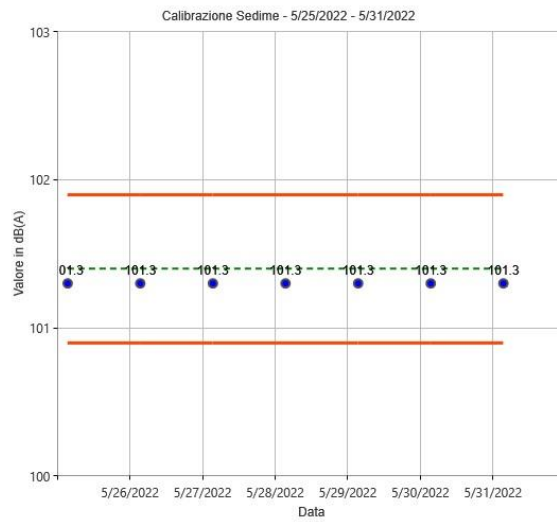
Figura 27: Calibrazioni check postazione Zona Militare Sedime
