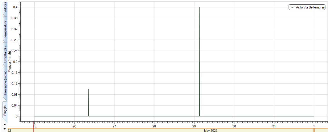
Figura 22: Grafico della pioggia acquisita dalla centralina Asilo Via Settembrini per il periodo 25 31 maggio 2022
